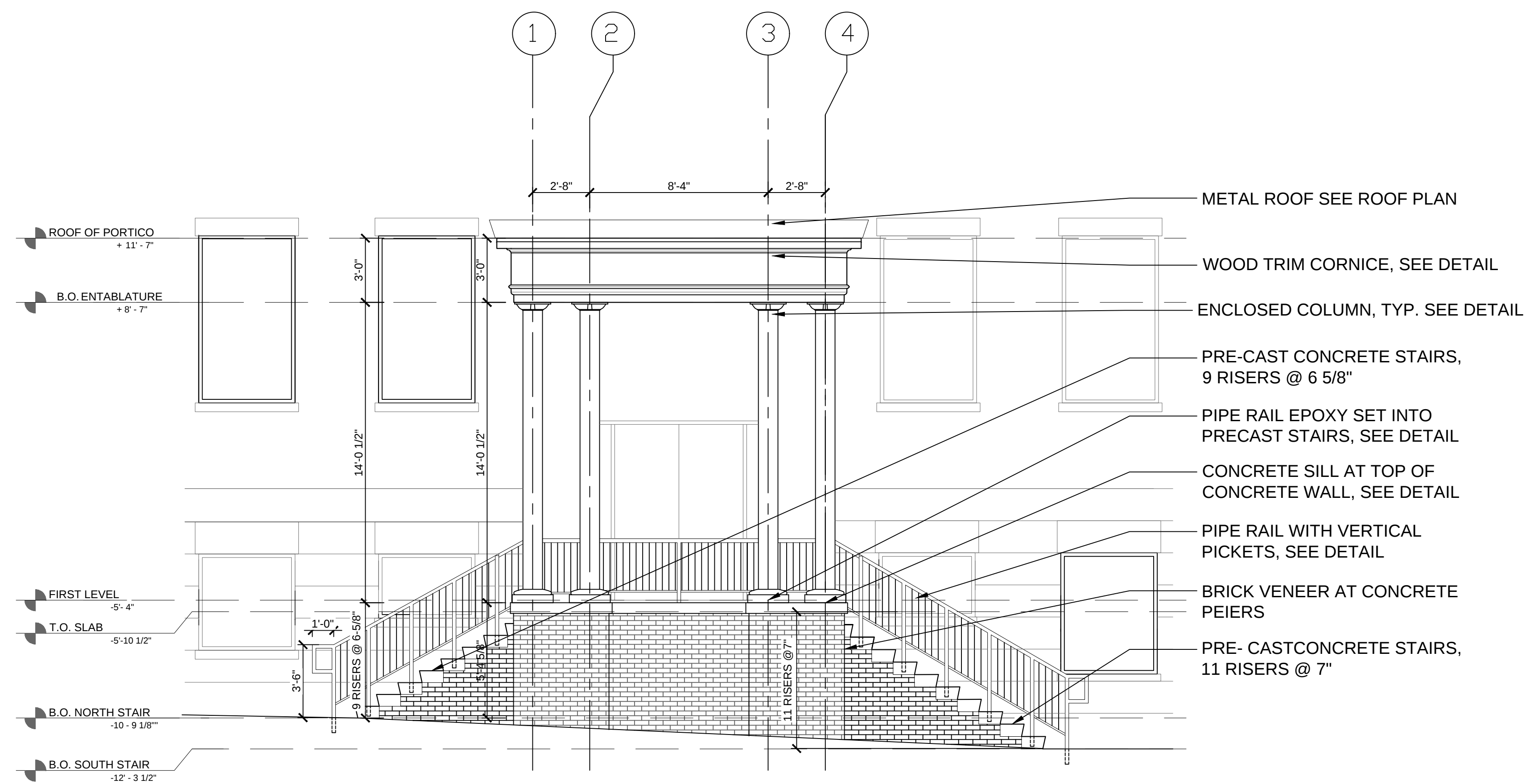
3 PORTICO NEW ELEVATION Scale: 1/4" = 1'-0"
