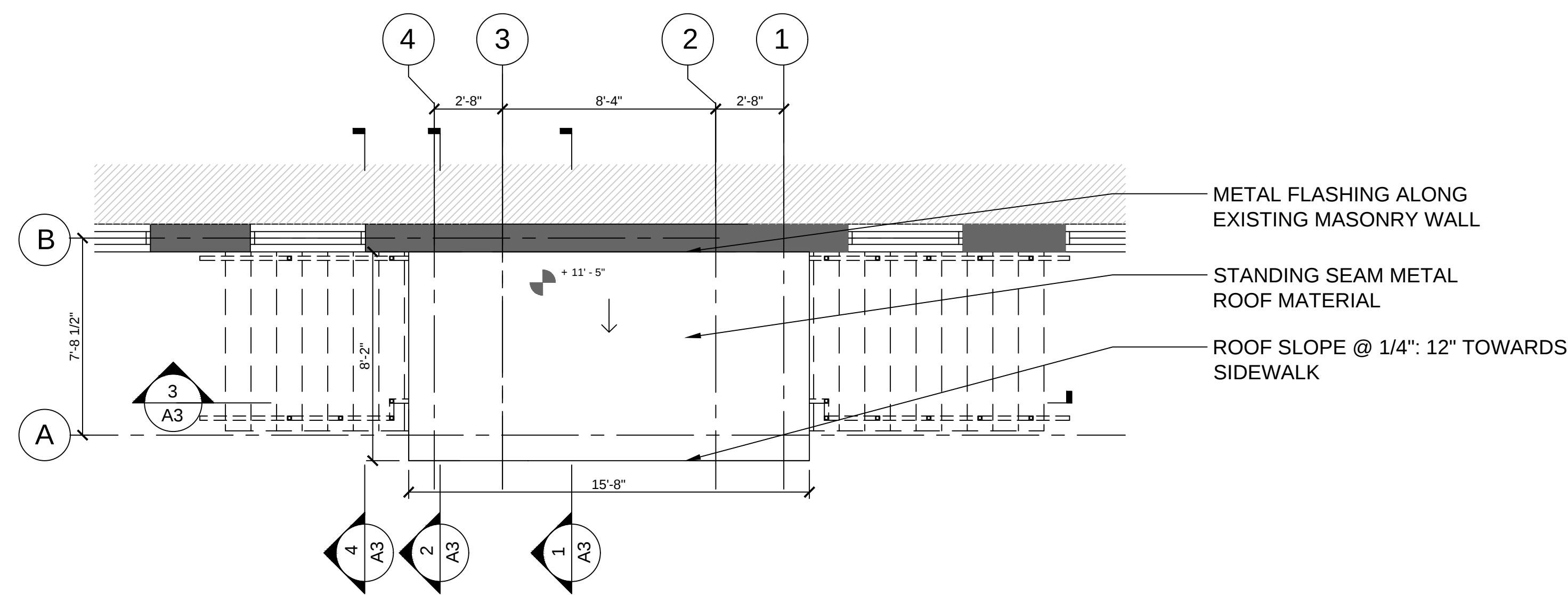
4 PORTICO ROOF PLAN Scale: 1/4" = 1'-0"
